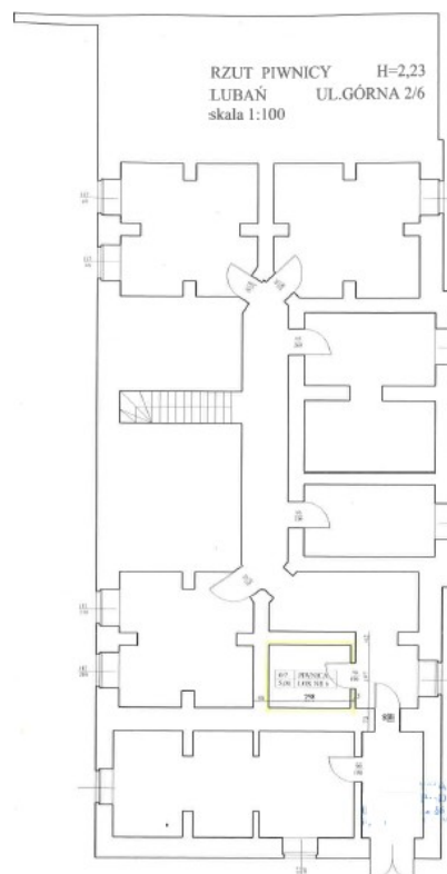
Rzut piwnicy
